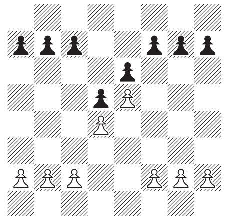
e5 Chain
