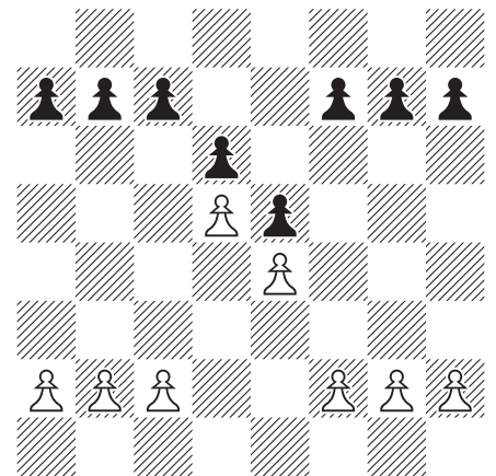
d5 Chain
